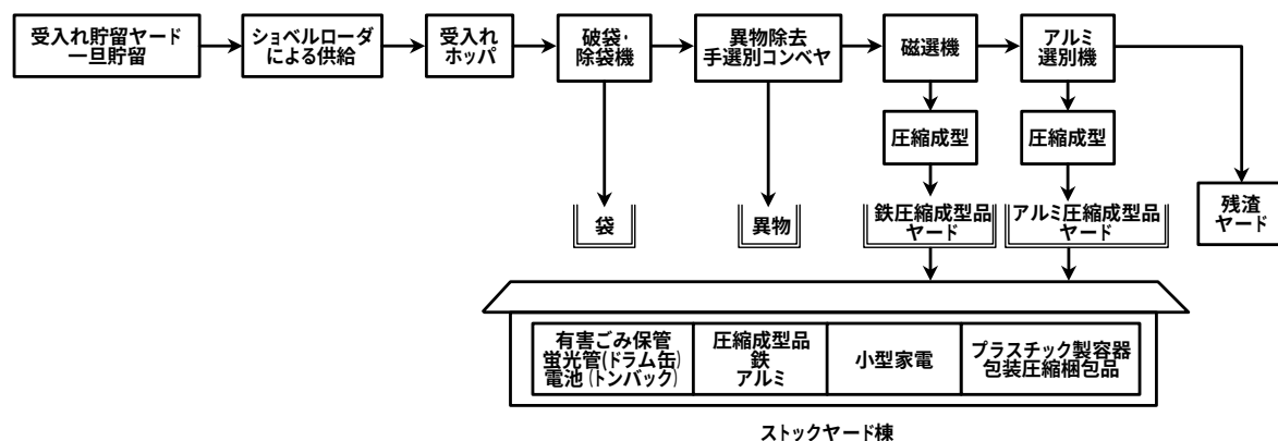
図 1.4.9 処理フロー(かん類)
