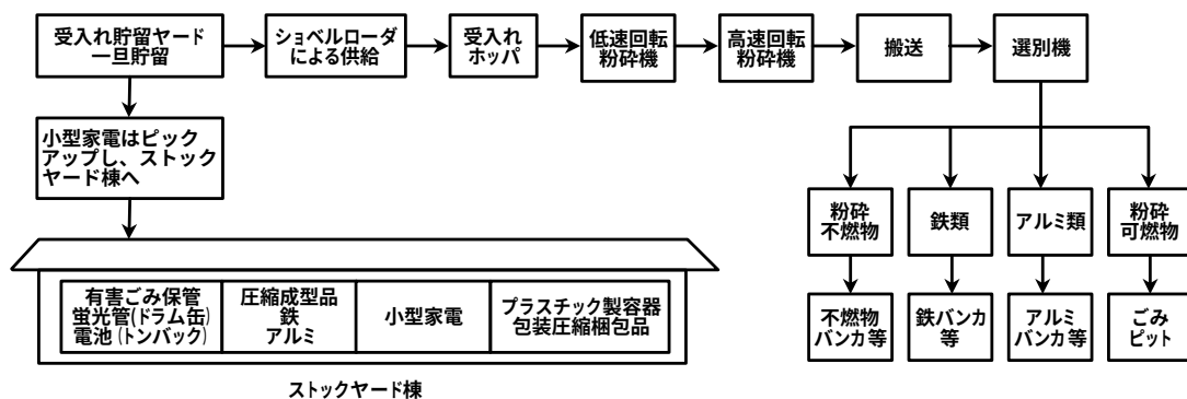
図 1.4.8 処理フロー(不燃ごみ・粗大ごみ)
