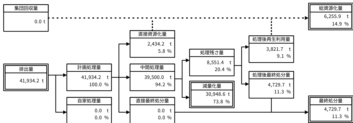
図 1.4.5(1) 一般廃棄物の処理状況フロー（現状）
