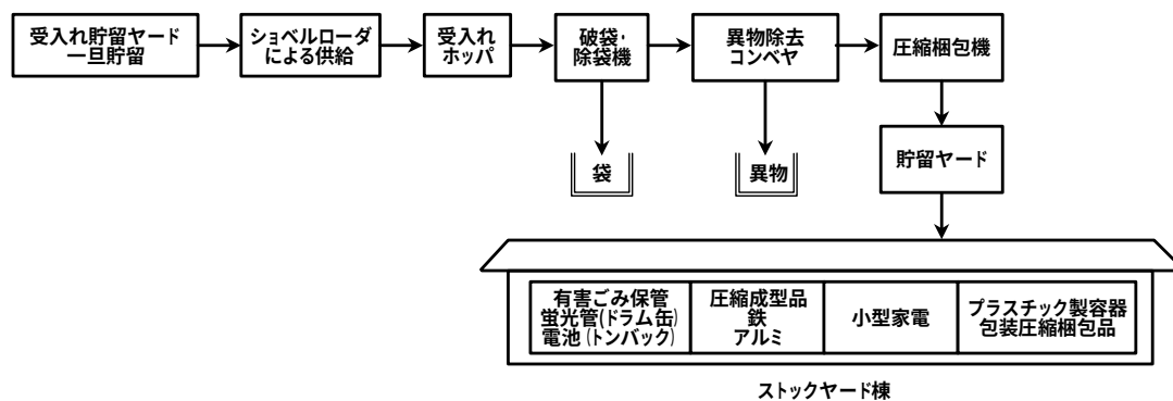
図 1.4.12 処理フロー(プラスチック製容器包装)
