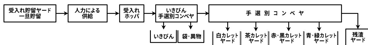
図 1.4.10 処理フロー(びん類)
