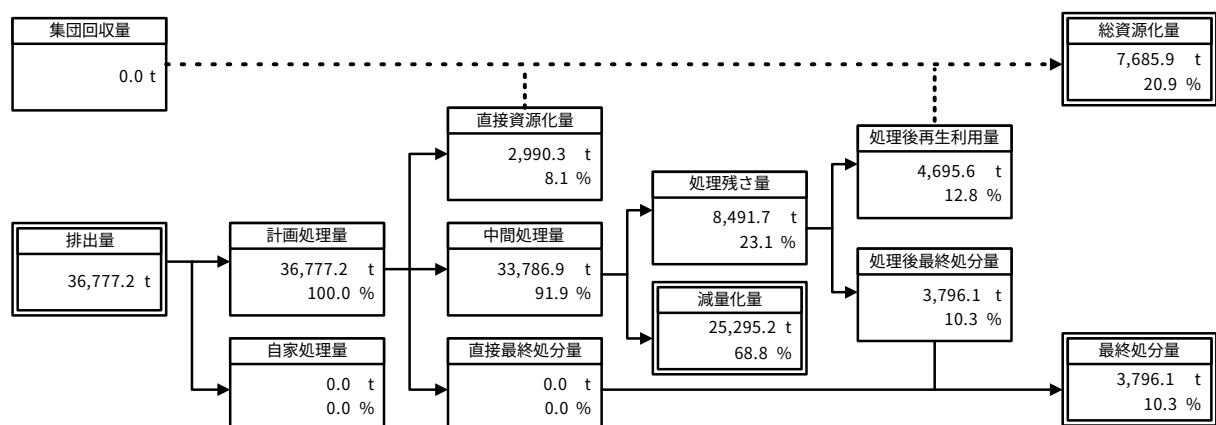
図 1.4.5(2) 一般廃棄物の処理状況フロー（目標達成時）
