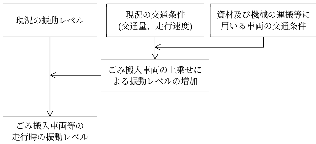
図 6.3.5 資材及び機械の運搬等に用いる車両の運行に伴う振動の予測手順
