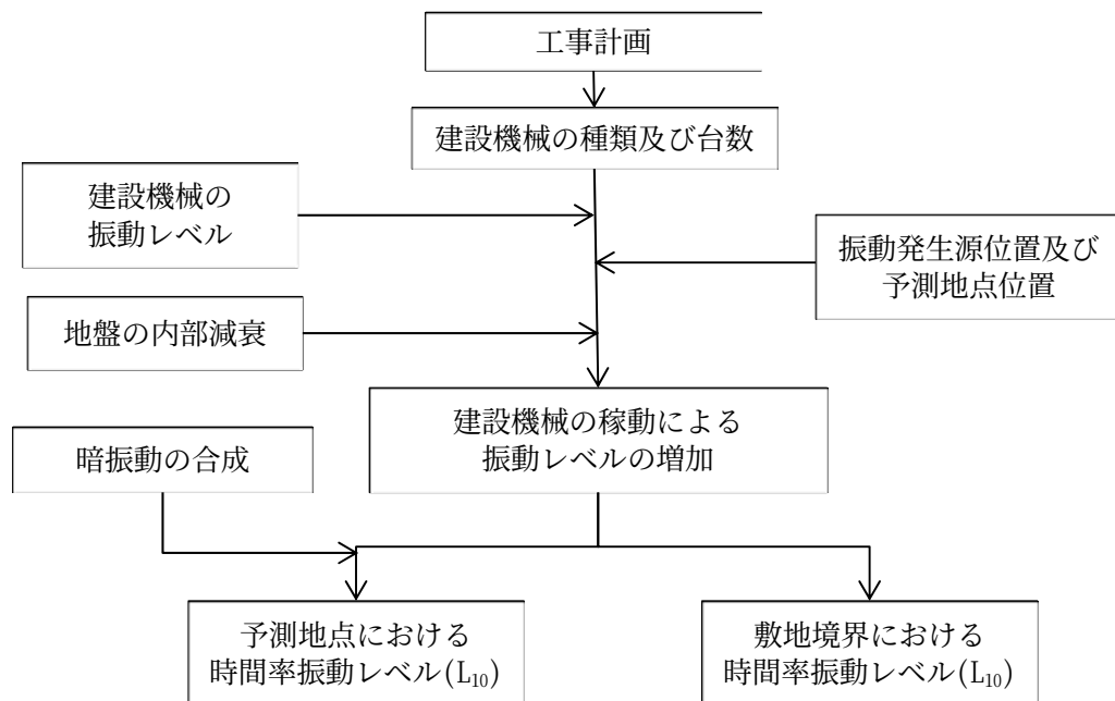
図 6.3.3 建設機械の稼動に伴う振動の予測手順
